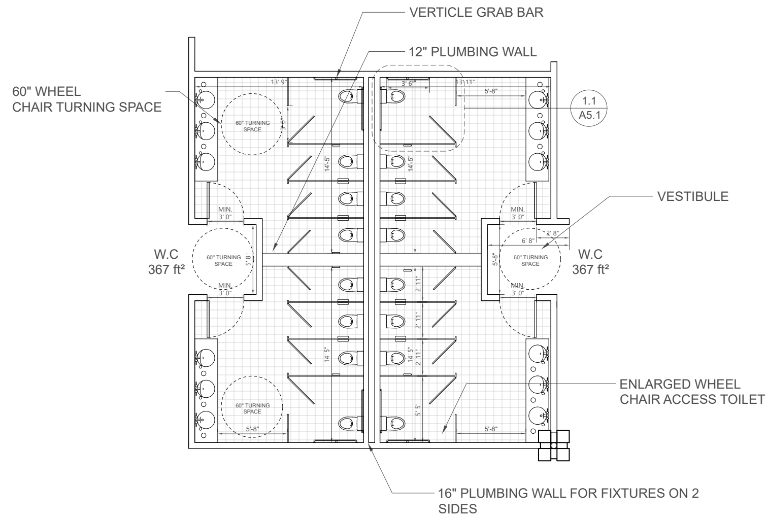
ADA BATHROOM SCALE: 1/8" = 1'-0"
