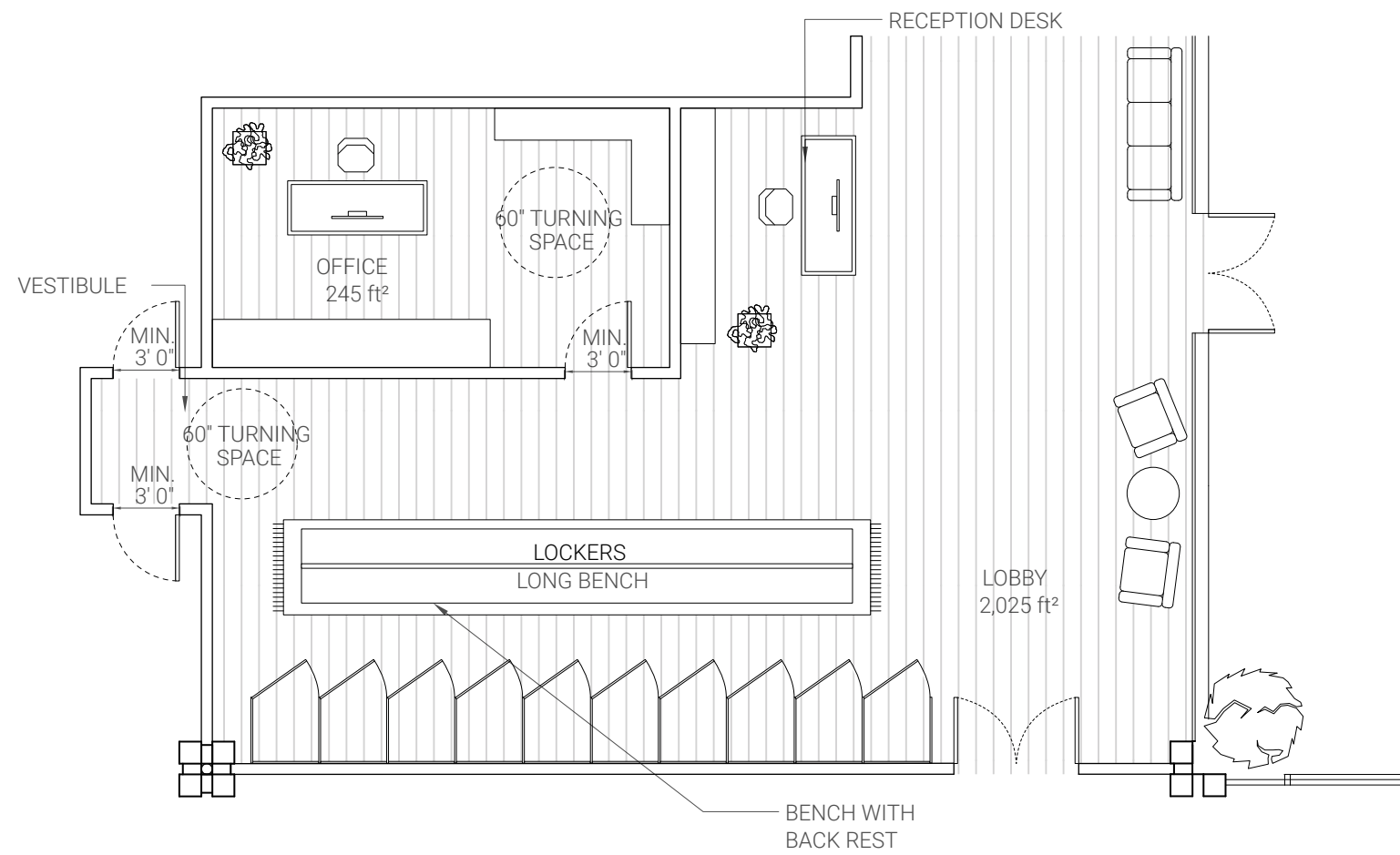
LOCKER ROOMS SCALE: 1/8" = 1'-0"
